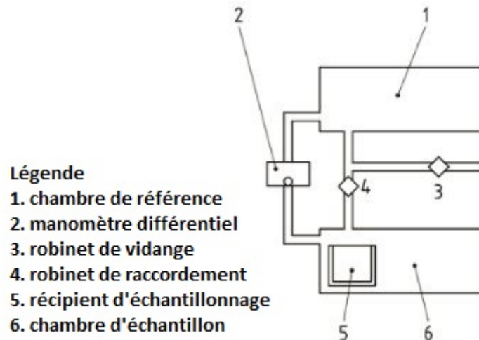
FIG. 51 Principe de mesure du pycnomètre [32]
