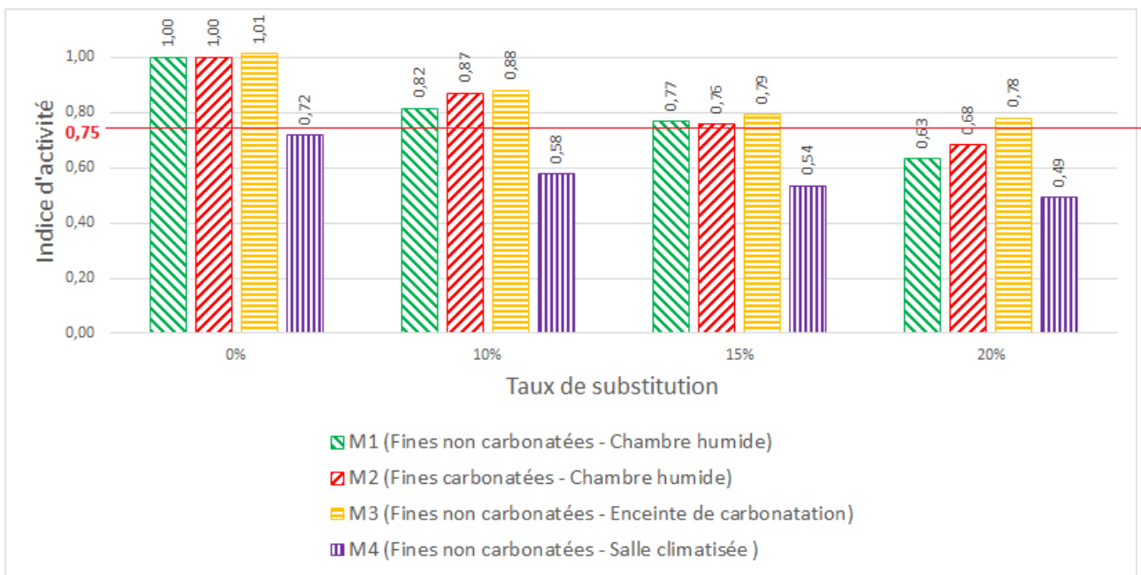
FIG. 85 Indice d'activité après 28 jours des mortiers à base de ciment substitué par des fines de fibres-ciment en fonction du taux de substitution et des conditions de cure
