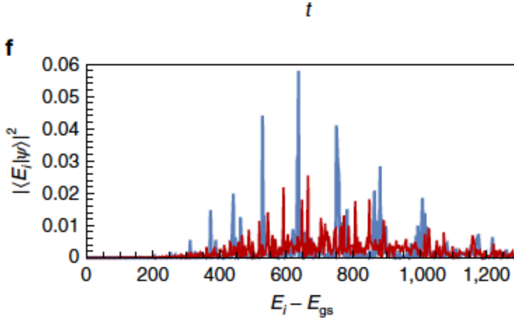
FIGURE 4.5 – Fonction d'autocorrélation en fonction de l'énergie pour un paquet d'onde gaussien lancé sur l'orbite périodique en bleu et à 45° de l'orbite périodique en rouge. Issu de [36]
