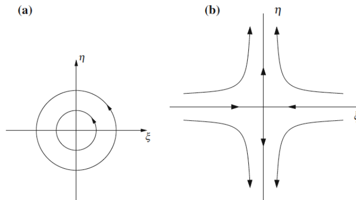
FIGURE 1.4 – a) Points fixes stables ou elliptiques b) points fixes instables ou hyperbolique Reproduit de [23]
