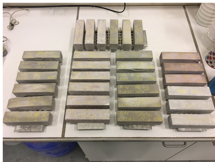
FIGURE 5 – Echantillons composés de sable et de fines de brique réalisés pour les essais d'attaque d'ions sulfate et de retrait
